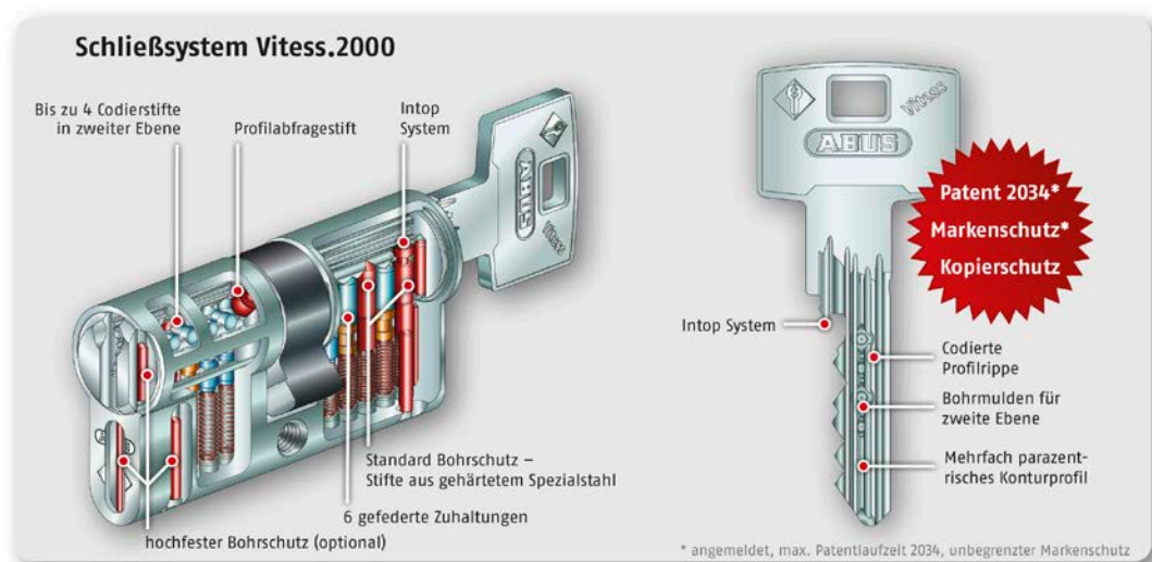
Abb. 1: Systemgrafik Vitesse.2000
